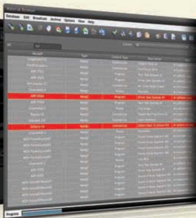
Material Browser
