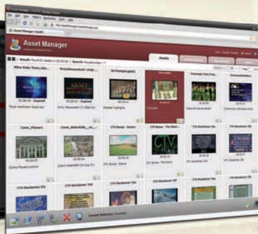
Web Interface
